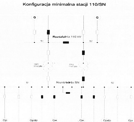
Rys.2. Konfiguracja minimalna GPZ/RPZ
