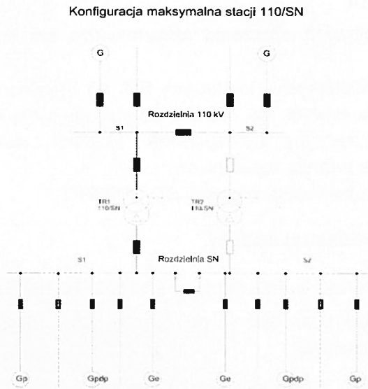
Rys.1. Konfiguracja maksymalna GPZ/RPZ
