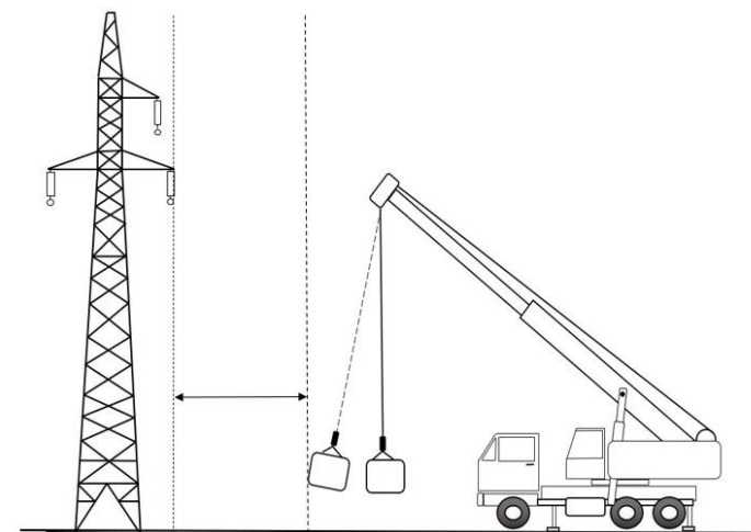
Rys 2. Odległość pozioma
