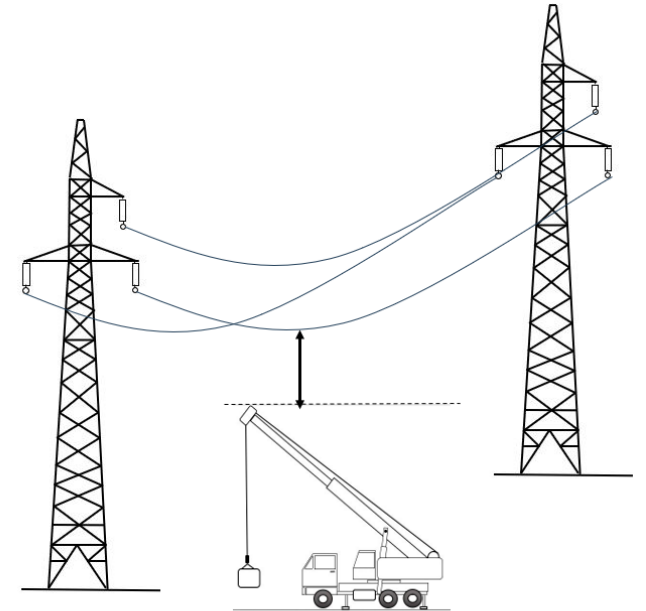
Rys 3. Odległość pionowa
