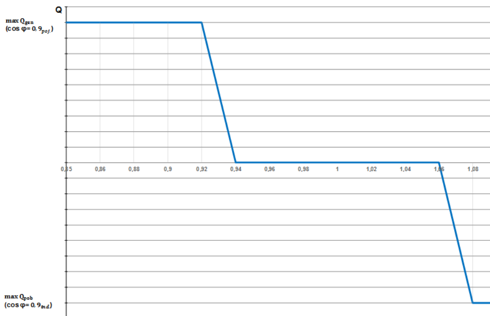
Rys. 3. Charakterystyka sterowania mocą bierną w funkcji napięcia wymagana przez TAURON Dystrybucja
