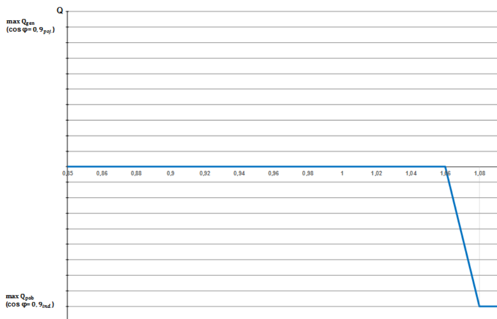
Rys. 4. Charakterystyka sterowania mocą bierną w funkcji napięcia dla falowników podłączonych jednofazowo, wymagana przez TAURON Dystrybucja
