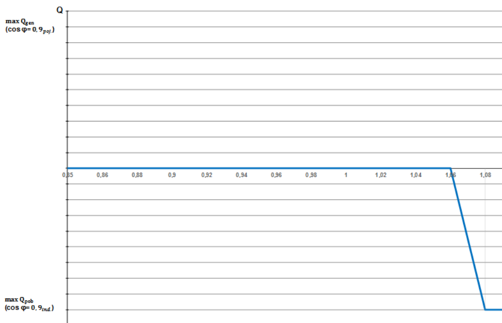
Rys. 4. Charakterystyka sterowania mocą bierną w funkcji napięcia dla mikroinstalacji podłączonych jednofazowo, wymagana przez TAURON Dystrybucja
