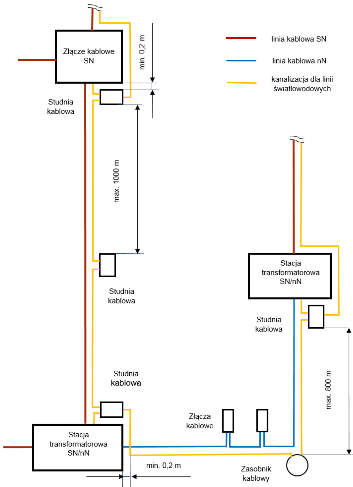
Rys. nr 3 Przykładowe rozmieszczenie sieci elektroenergetycznej i kanalizacji światłowodowej.
