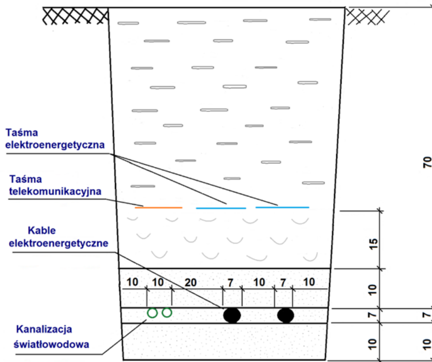
Rys. nr 1 Poziome rozmieszczenie dwóch kabli elektroenergetycznych nN i kanalizacji światłowodowej.
