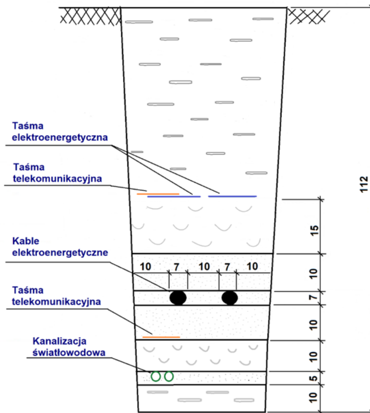
Rys. nr 2 Pionowe rozmieszczenie dwóch kabli elektroenergetycznych nN i kanalizacji światłowodowej.
