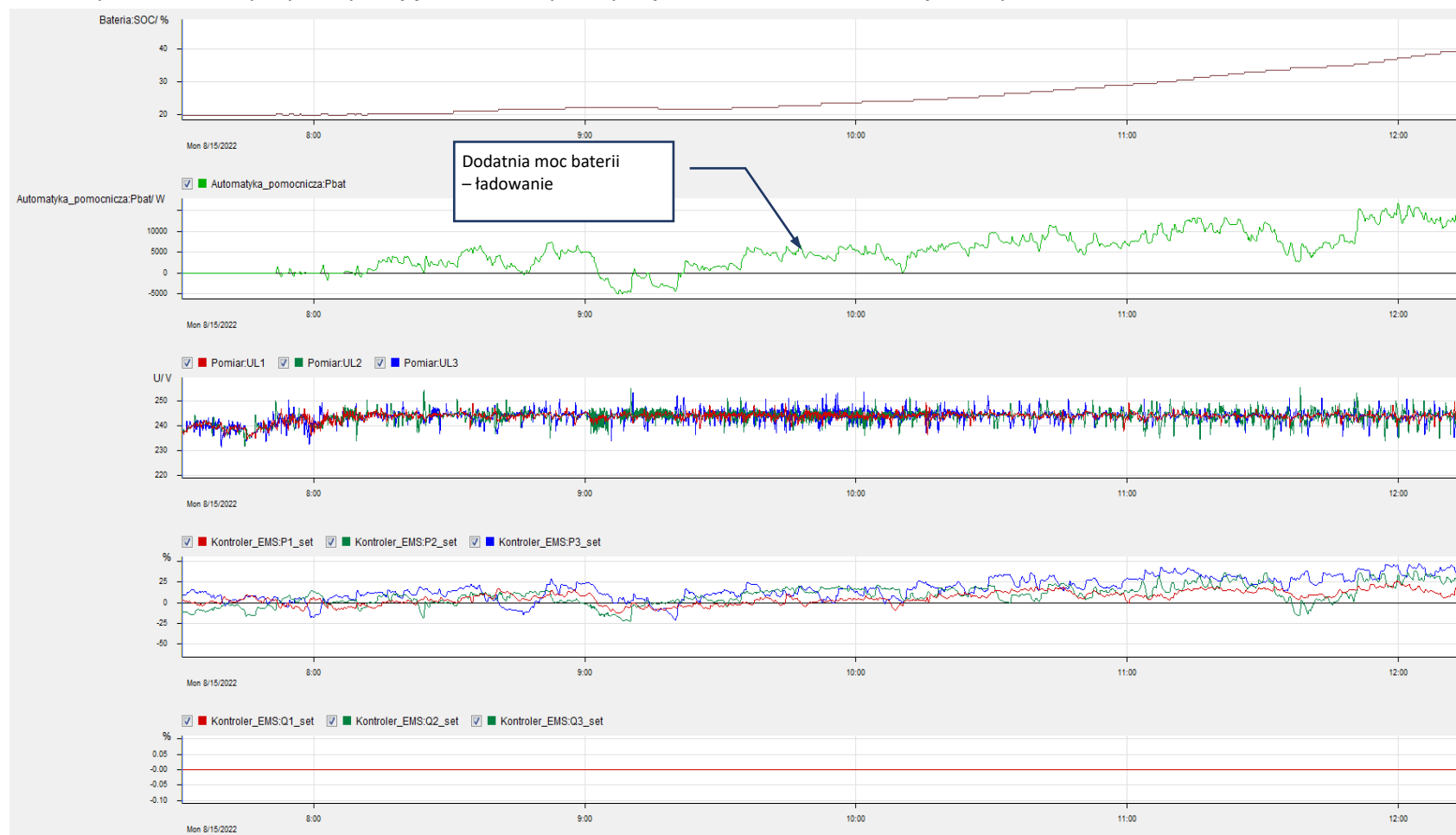
Obniżanie napięcia mocą czynną – fragment rejestracji dobowej z 15-08-2022
